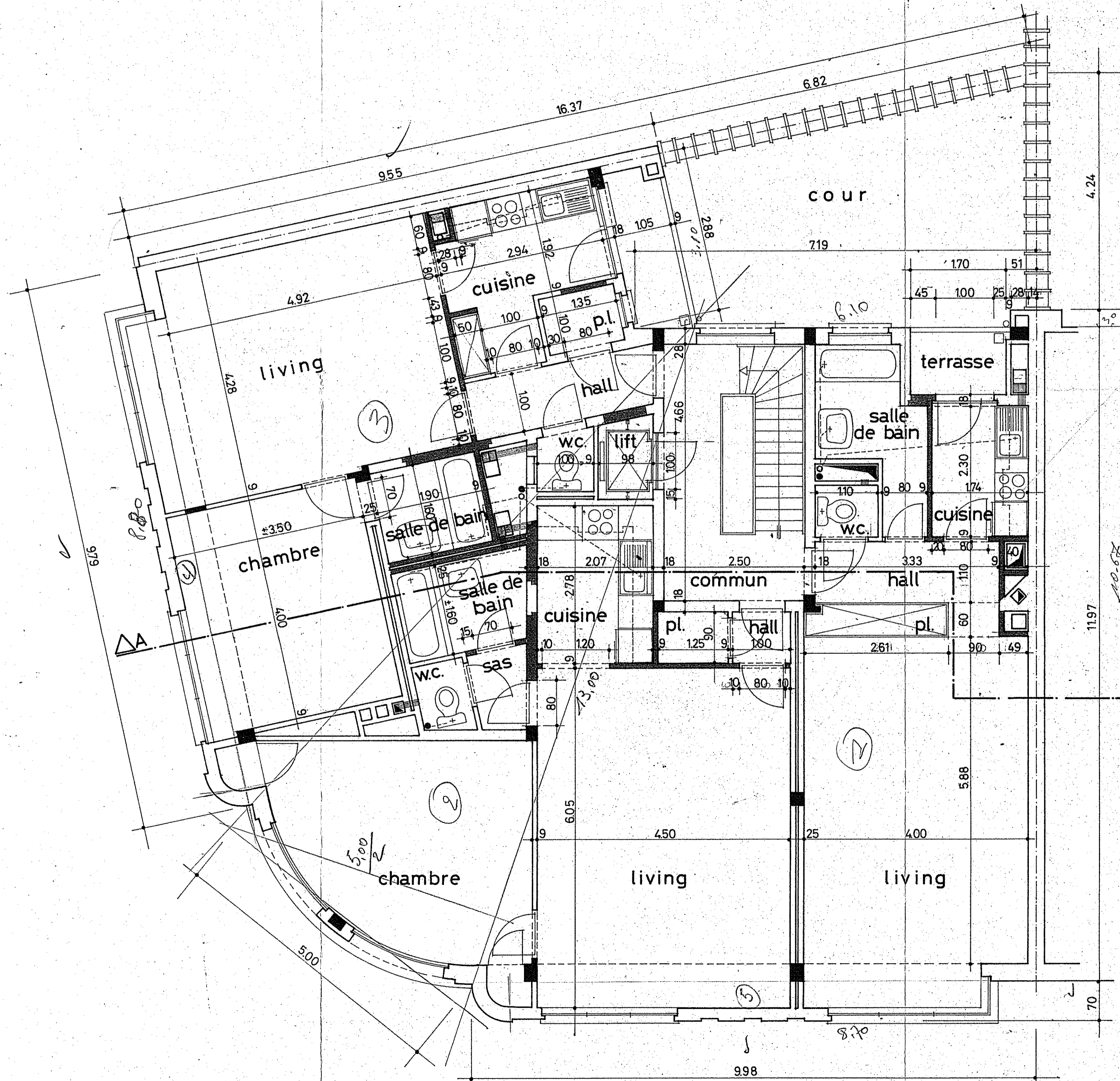
plan étages 1,2,3,4,5 nouvelle situation
